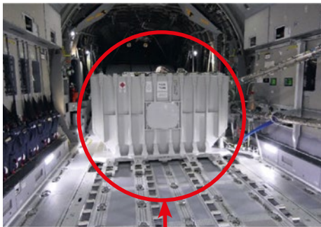
2x 5000kg Zusattank im Laderaum
