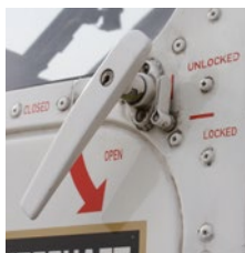
Öffnen der Cockpittüren (rechts u. links)
